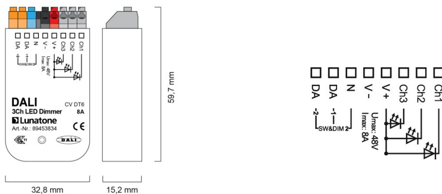
Geometrie Dose Version 8A Art.Nr.: 89453834 Version 4A Art. Nr.: 89453828
