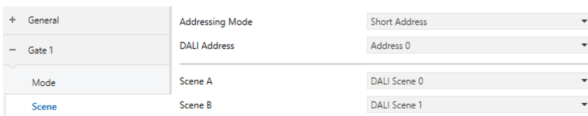
Abb.12 Gate Einstellungen ETS: Beispiel Standard Scene Gate
