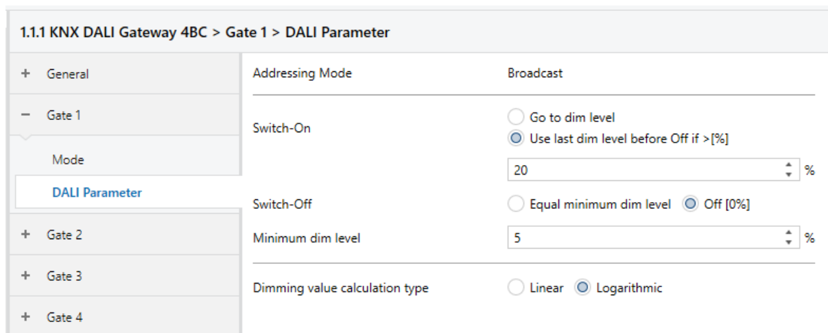
Abb.6 Gate Einstellungen ETS: DALI Parameter
