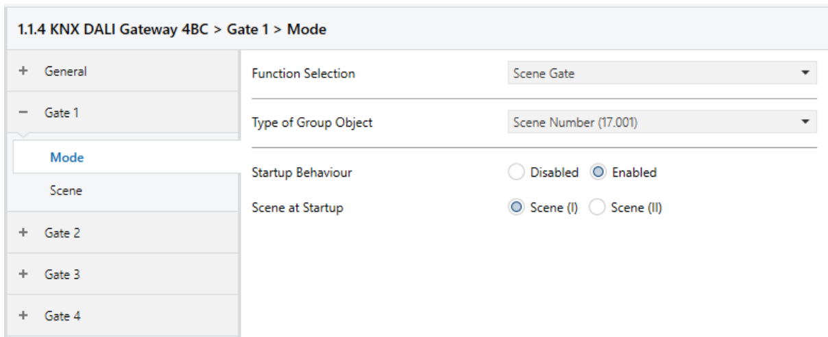
Abb.11 Gate Einstellungen ETS: Beispiel Standard Scene Gate
