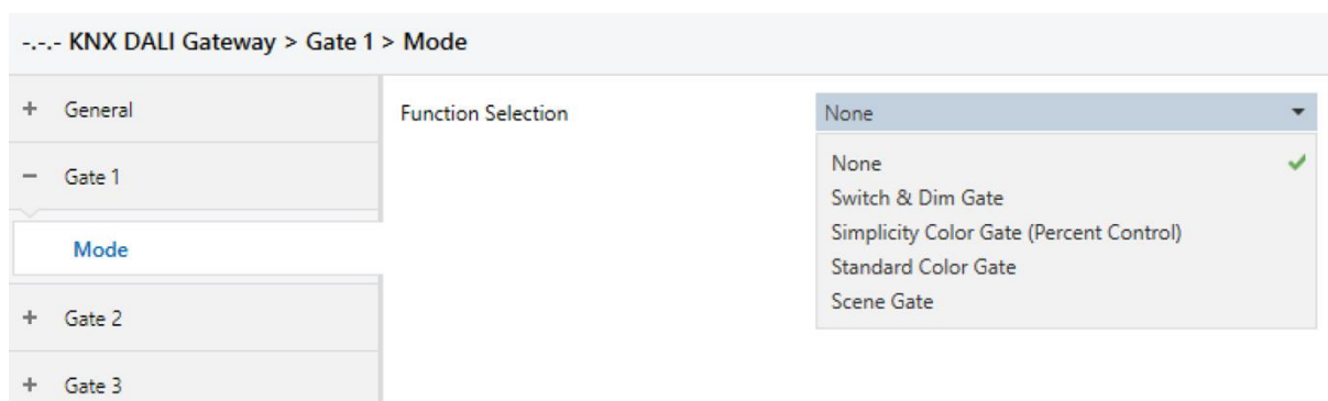
Abb.5 Gate Einstellungen ETS: Gate Type auswählen
