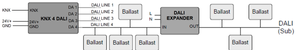
Abb. 2 Installationsbeispiel, Erweiterung mittels DALI Expander (Art. Nr. 89453847)
