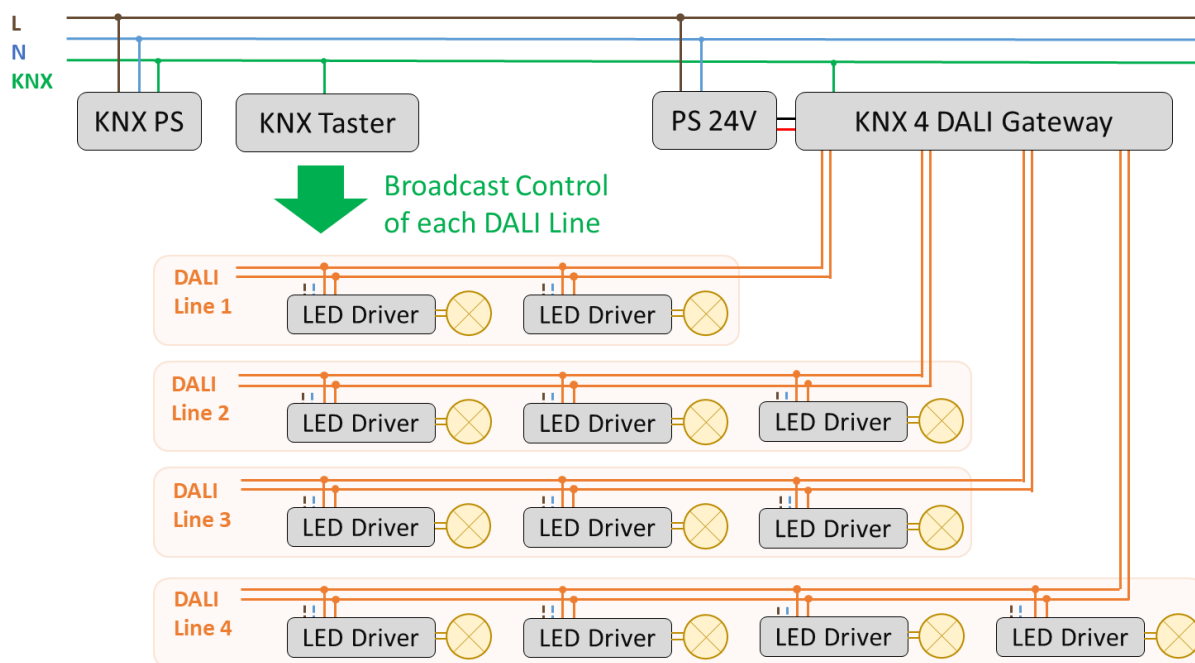
Abb.4 Beispiel KNX System mit KNX 4 DALI Gateway und 4 DALI Linien
